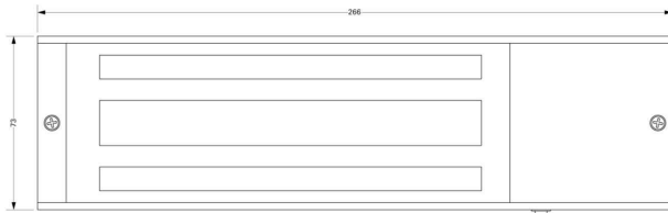
Armlock 281-005
