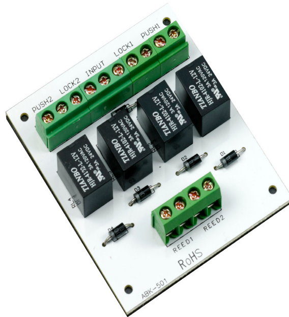
Door Interlock Module
