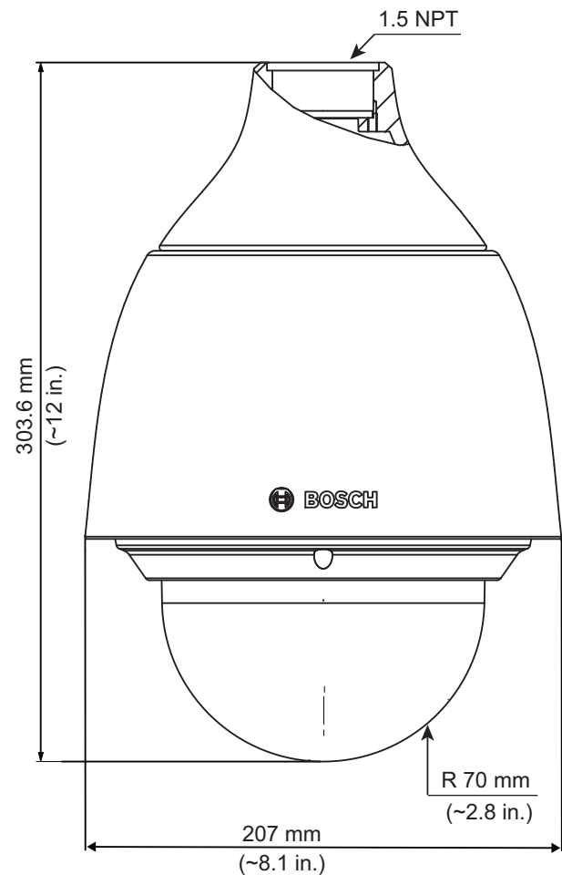
Fig. 5: Pendant model
